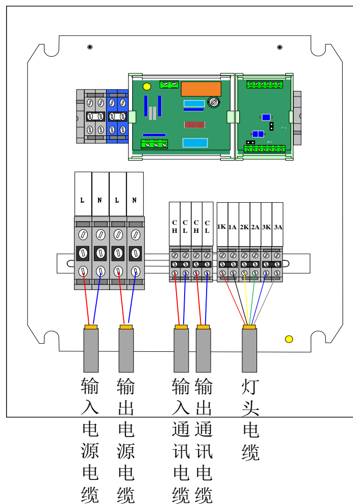
图 22 电缆接头制作及电缆与接地线的连接方法
