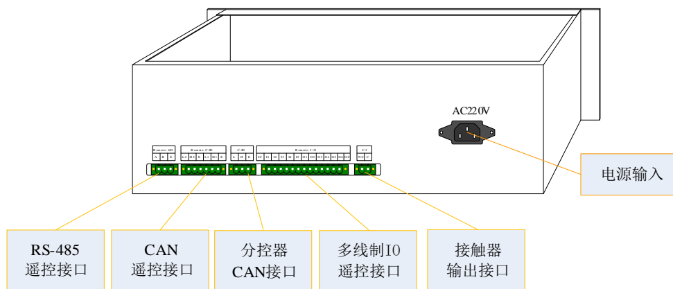
图 5 主控制器后面元件布置
