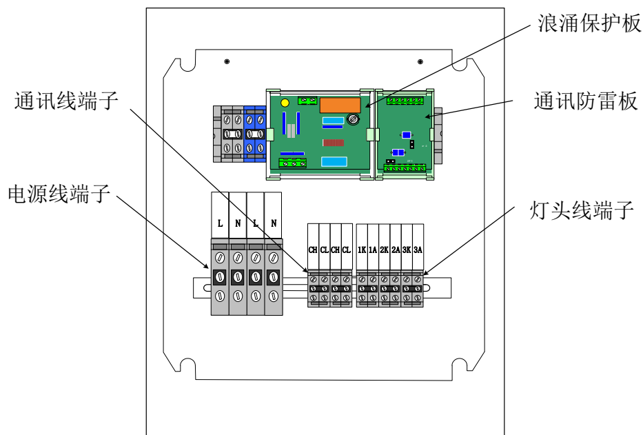
图 8 分控箱内部元件布置
