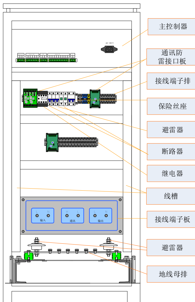
图 3 主控制柜内部后面元件布置
