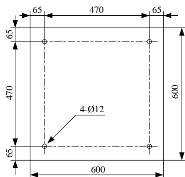
图9 控制柜底座尺寸
