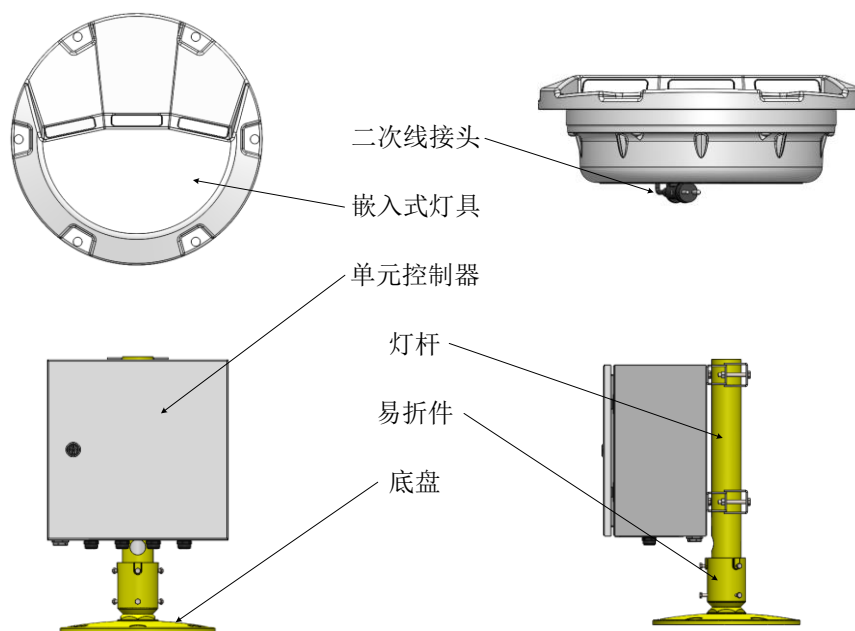
图6 立式灯具外观
