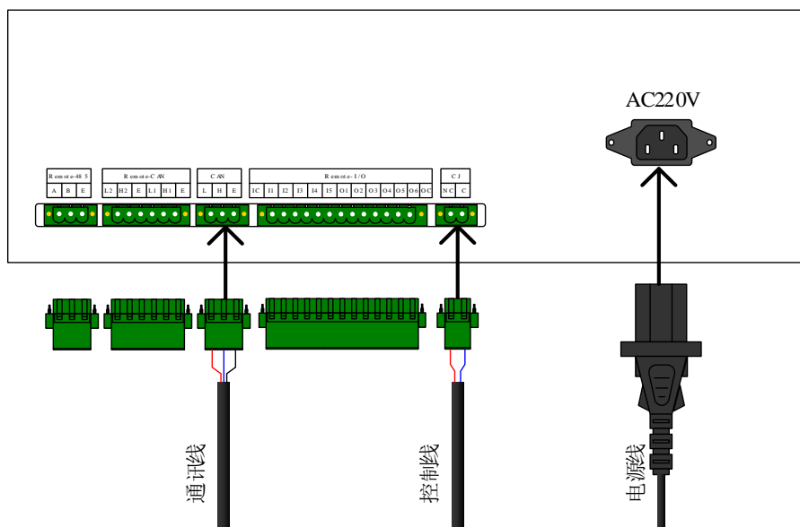
图 18 控制器基本接线
