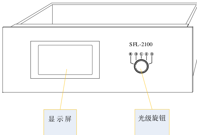
图 4 主控制器正面元件布置
