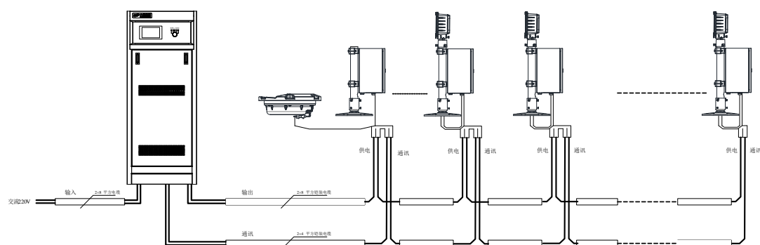
图 25 闪光灯系统示意图
