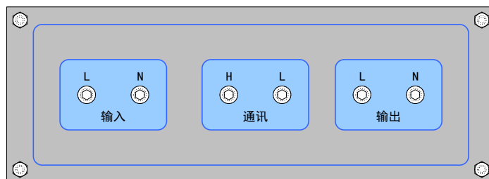
图 16 控制柜接线端子板
