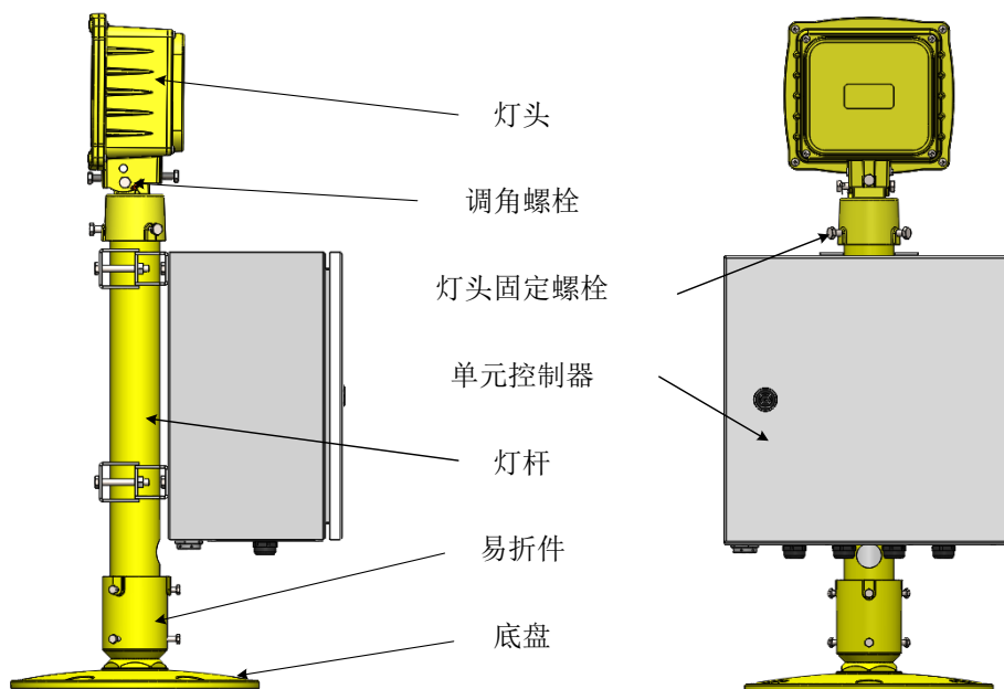
图6 立式灯具外观
