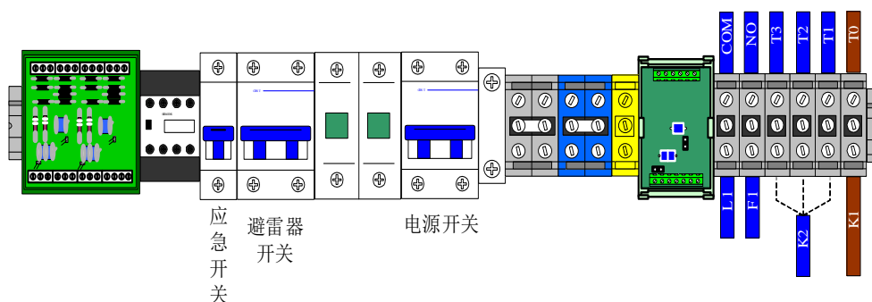
图 17 控制柜端子排
