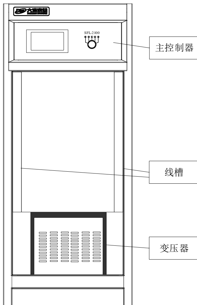
图2 主控制柜内部前面元件布置
