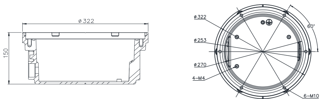
图8 嵌入式灯具底座图
