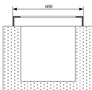
图10 控制柜安装基础截面图
