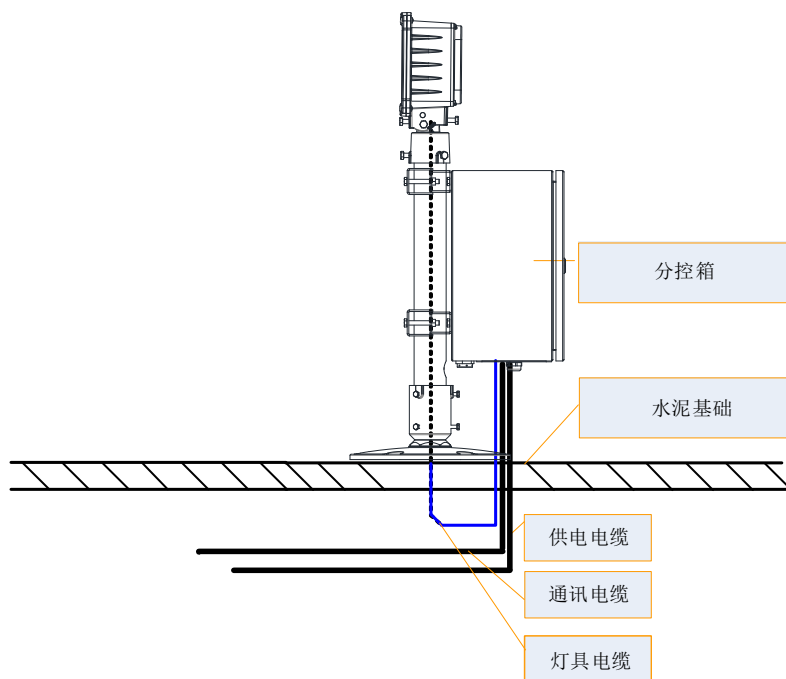
图9 立式灯具一体安装示意图
