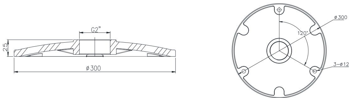
图7 立式灯具底座图
