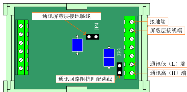
图 23 通讯接口板示意图
