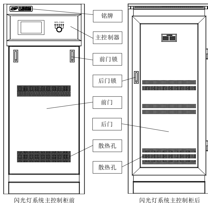
图 1 闪光灯系统主控制柜外观
