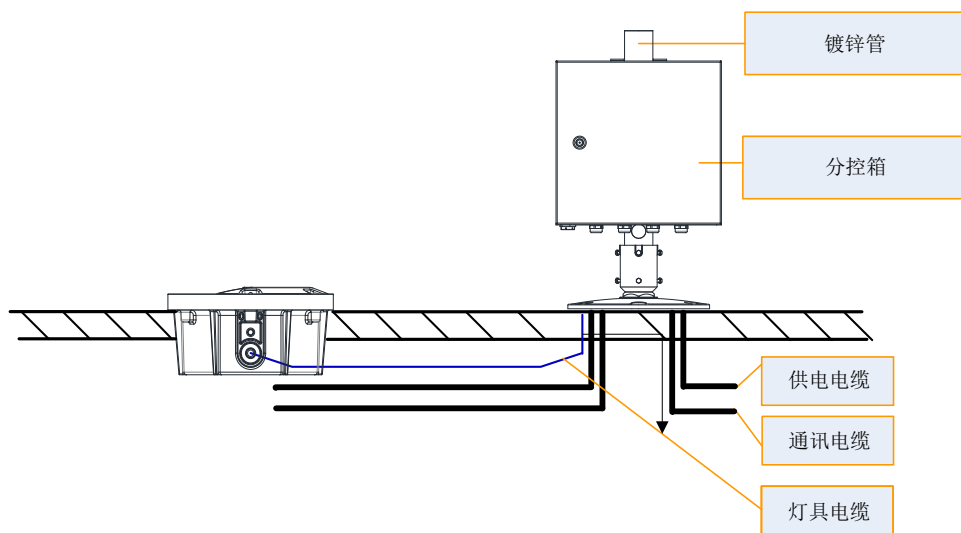
图 15 嵌入式灯具分体安装示意图
