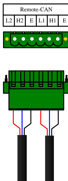
图 19 遥控 CAN 网络接线
